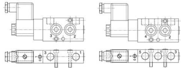
Abb. 2: Anschluss 8500N
